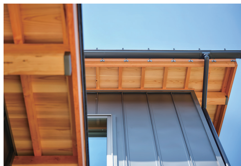
木造らしさを表現できる化粧垂木の軒裏
